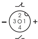
Цоколевка соединителя CS S261-3 (вид со стороны монтажа)
